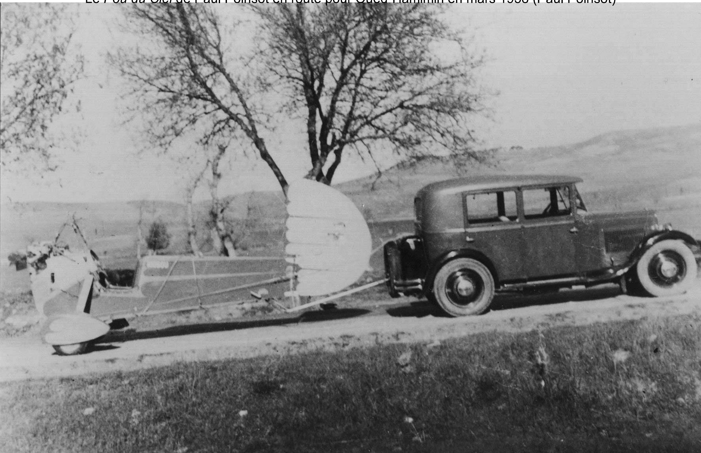
Le Pou du Ciel de Paul Poinot en route pour Oued-Hamimin en mars 1938 (Paul Poinot)
